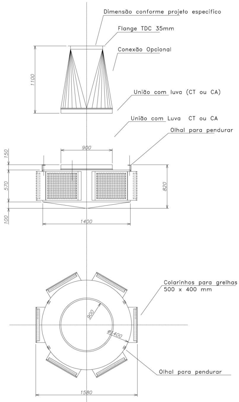
CAIXA DIFUSORA DE AR PARA 06 GRELHAS PADRÃO REFRIN
