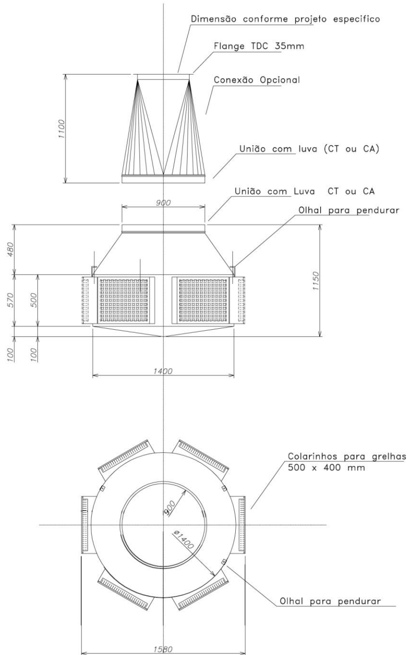
CAIXA DIFUSORA DE AR PARA 06 GRELHAS PADRÃO REFRIN
