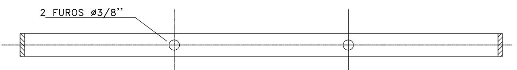
SUPOORTE INTERNO PARA DUTO GIROVAL LADO MAIOR DE 813mm A 1950mm
